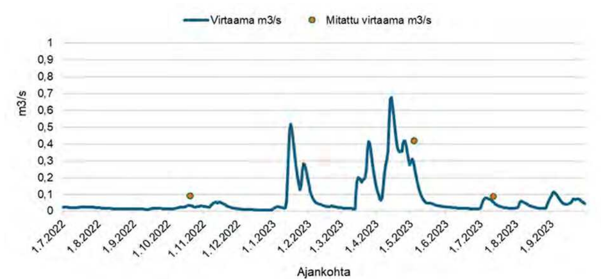
Kuva 2. Koivusillanjoen simuloitu ja mitattu virtaama (1.7.2022–30.9.2023) Koivusillanjoen alaosalla. Mittaukset tehtiin vesinäytteenottojen yhteydessä. Simulointi: Ympäristöhallinnon Vemala WSFS-vesistömallijärjestelmä. Lähde Holmberg ym. 2023.
